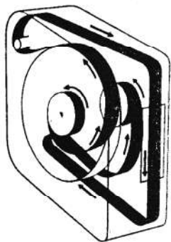
Filmens løb i super-8 kassetten.
